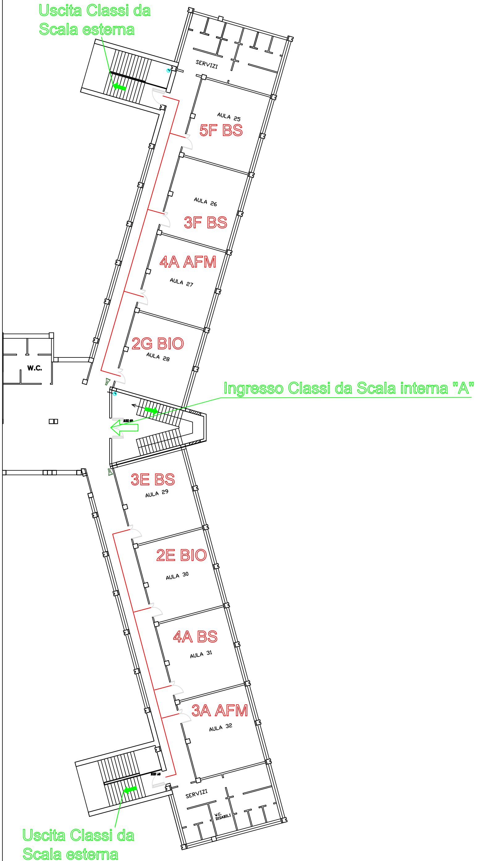
IT DELEDDA - SEZIONE STACCATA C/O IISS "GALILEI-COSTA-SCARAMBONE" - PIAZZA PALIO - LECCE - PIANO SECONDO
